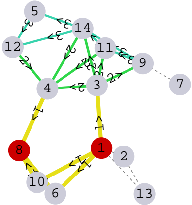
layer 3
