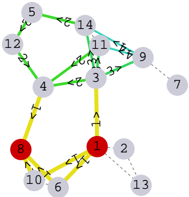
layer 4
