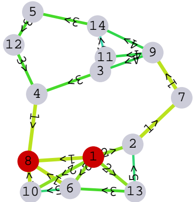
layer 6
