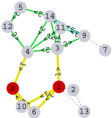
layer 3
