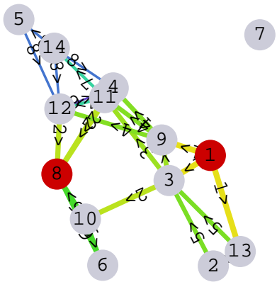
layer 9
